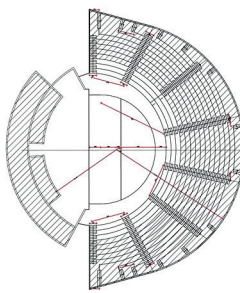
ΘΕΑΤΡΟ (Κλίμακα 1:500)
